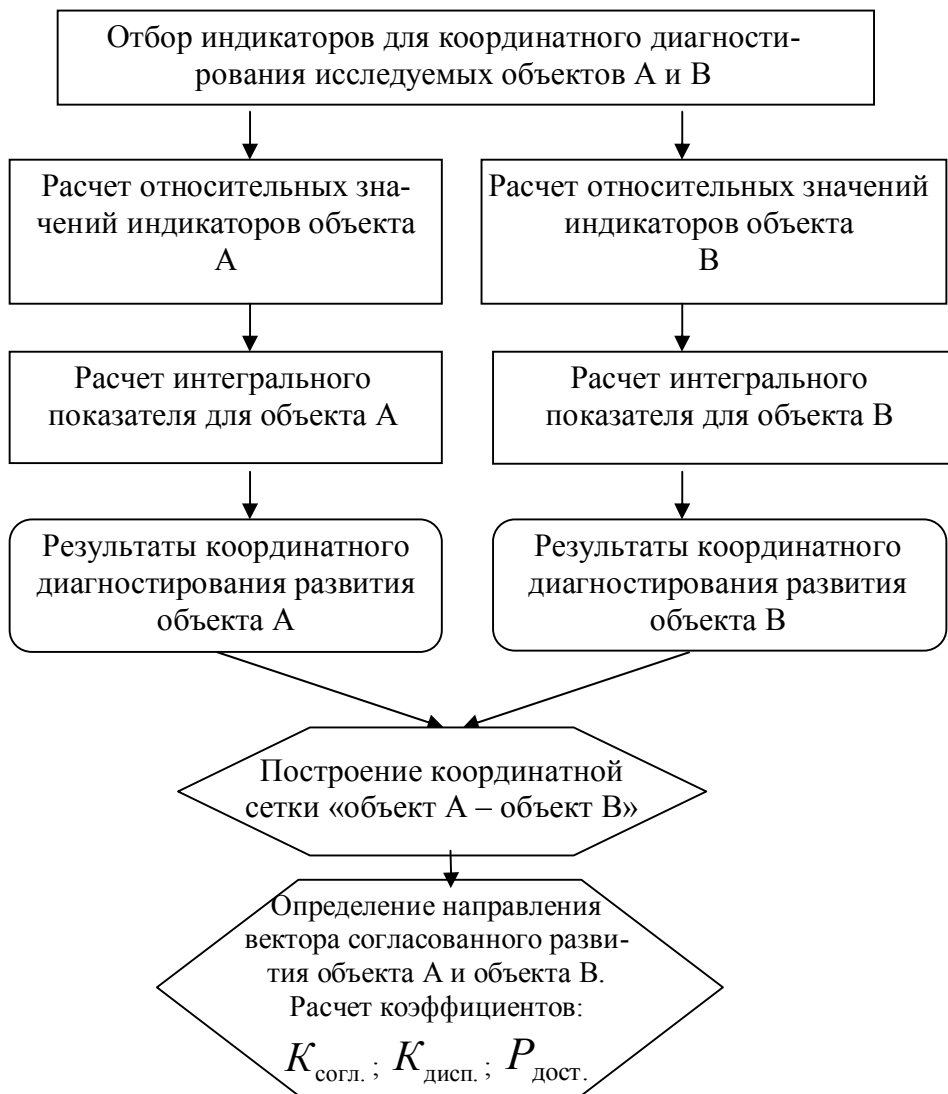
Рис.1. Алгоритм координатного диагностирования
